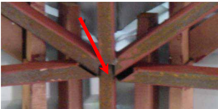
Onvolledig laswerk van een kapconstructie
